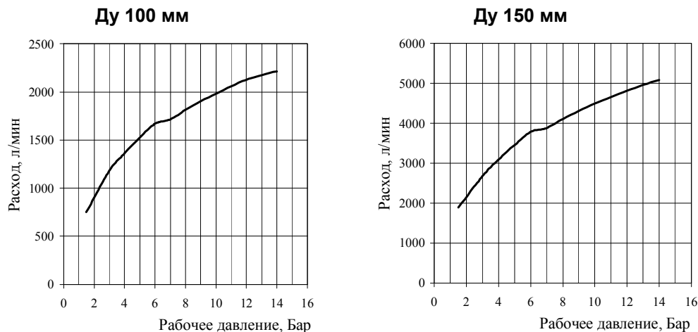
Рис. 4а. Диаграммы зависимости давления от расхода
