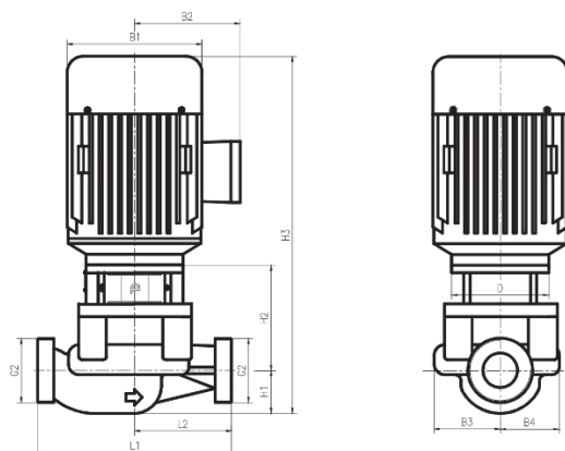
Рис. 20а. Габаритно-присоединительные размеры модели TD32-6(l)/2
