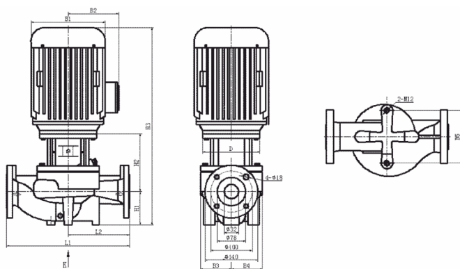
Рис. 206. Габаритно-присоединительные размеры модели TD32-10(I)/2
