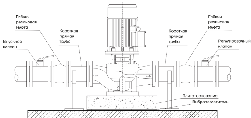
Рис. 14 Схема подключения насоса
