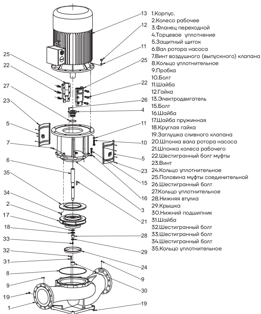
Рис. 18-В TD200-TD250
