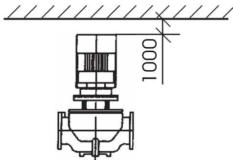
Рис. 10 Электродвигатель > 5 кВт
